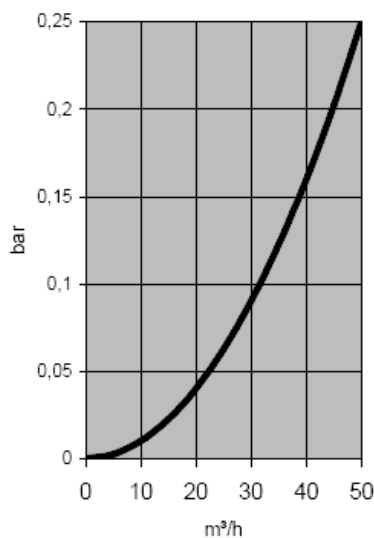
Référence A-TF30-025 pour bouteille 30"
