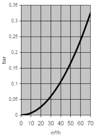
Référence A-TF42-025 pour bouteille 42"
