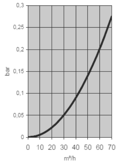
Courbes de perte de charge
