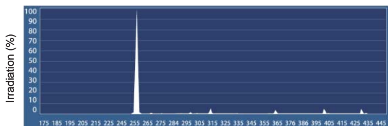
SPECTRE D'EMISSION DES LAMPES GERMICIDES
