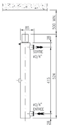
UV405
